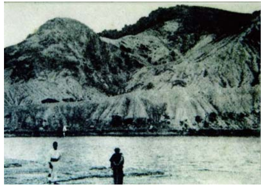
写真2 写真3の右奥にある山を背景にして火口底で撮影
