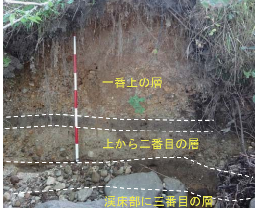
安達太良山の西麓に見られる火山泥流堆積物
