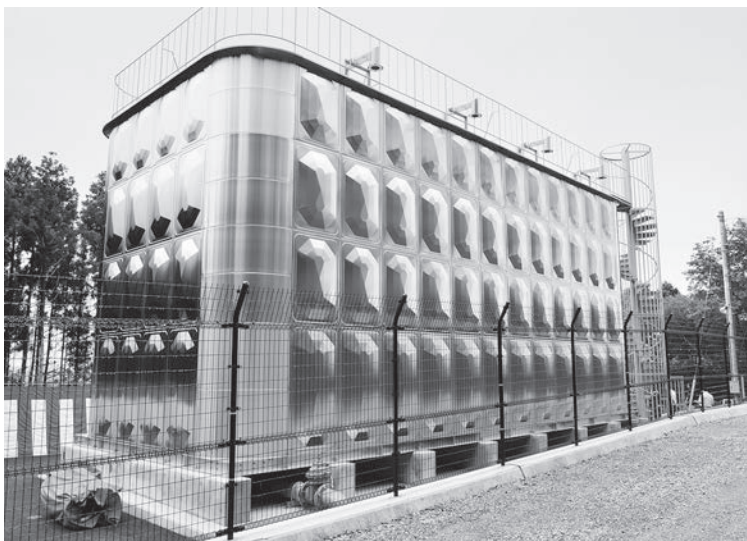
▲ステンレス製で容量が500立方メートルの高松配水場
